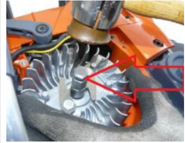
40000308 Schwungradwerkzeug
