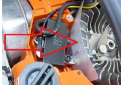
40028059 Einstellscheibe Zündspalt
